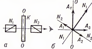
Рис. 3. Схема наблюдения интерференции поляризованных лучей (хроматической поляризации) в параллельном световом потоке. Поляризатор N_1 пропускает лишь одну линейно поляризованную (в направлении N_1N_1 ) составляющую исходного пучка. В пластинке K , вырезанной из двулучепреломляющего одноосного кристалла параллельно его оптической оси OO и установленной перпендикулярно пучку, плоскополяризованный луч разделяется на составляющую A_e с колебаниями электрического вектора, параллельными OO (необыкновенный луч), и составляющую A_o , колебания электрического вектора к-рой перпендикулярны OO (обыкновенный луч). Показатели преломления материала пластинки K для этих двух лучей ( n_e и n_o ) различны, а следовательно, различные скорости их распространения в K , вследствие чего эти лучи, распространяясь по одному направлению, приобретают разность хода. Разность фаз их колебаний при выходе из K равна \delta = (1/\lambda) \cdot 2\pi l(n_e - n_o) , где l — толщина K , \lambda — длина волны падающего света. Анализатор N_2 пропускает из каждого луча только его слагающую с колебаниями, лежащими в плоскости его главного сечения N_2N_2 . Если N_1 \perp N_2 (оптические оси анализатора и поляризатора скрещены), амплитуды слагающих A_1 и A_2 равны, а разность их фаз \Delta = \delta + \pi . Они когерентны и интерферируют между собой. В зависимости от величины \Delta на к.-л. участке пластинки K наблюдатель увидит этот участок тёмным [ \Delta = (2k + 1)\pi , k — целое число] или светлым ( \Delta = 2k\pi ) в монохроматическом свете и окрашенным — в белом свете.
